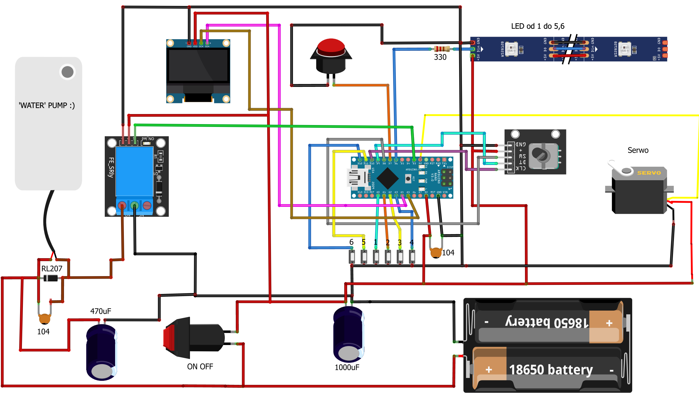
Jako zasilanie używam modułu zasilania awaryjnego mini UPS na 2x18650, 5V, USB-C.
